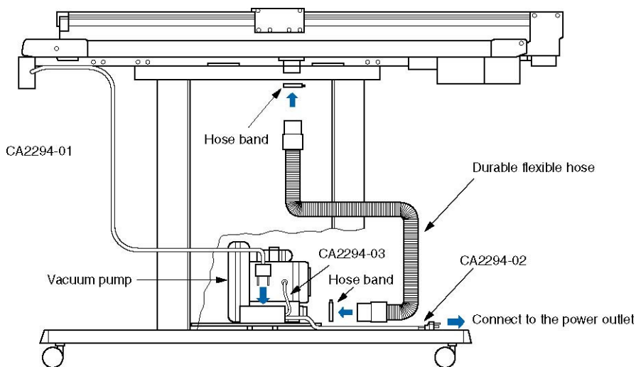
機器配置圖 - 真空泵(Vacuum pump)為選購品
